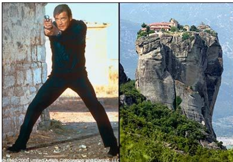
Εικόνα 3: Τα μετέωρα χρησιμοποιήθηκαν ως τόπος γυρισμάτων της ταινίας του James Bond με τίτλο For your Eyes Only .
